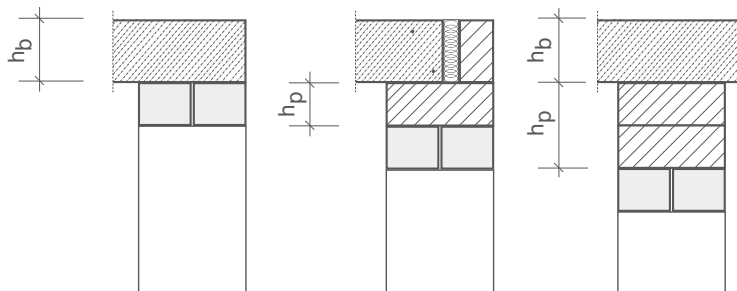
Schnitt A-A (Varianten der Druckzone)
